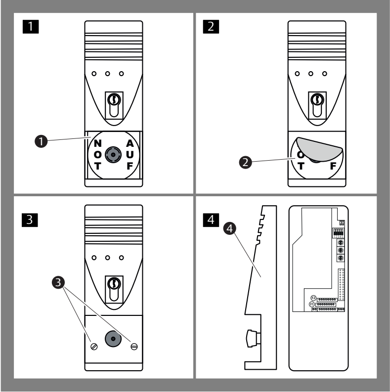
Abb. 3: Gehäuse öffnen
