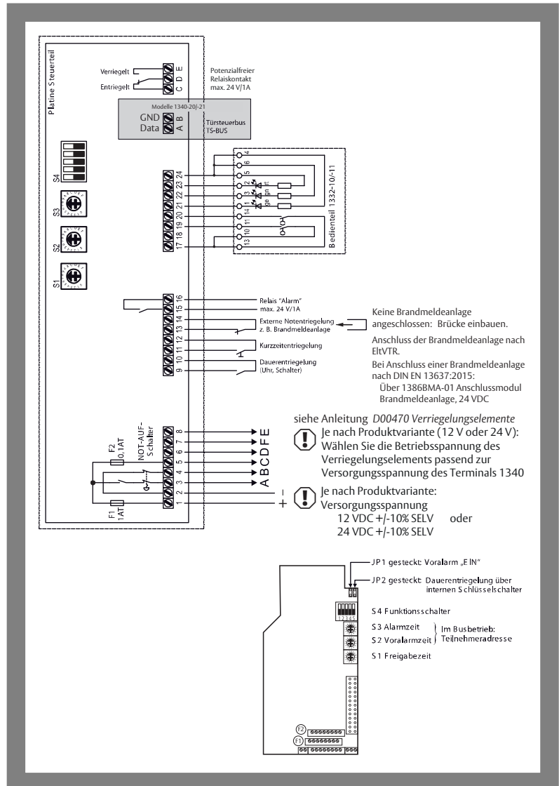
Abb. 6: Anschlussplan
