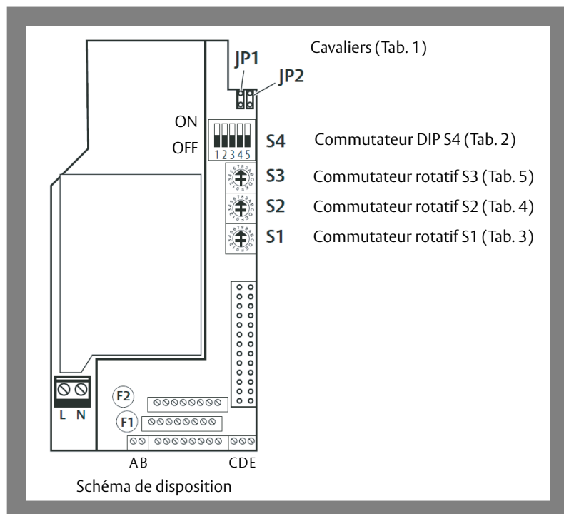
Fig. 7: Commutateurs et raccords
