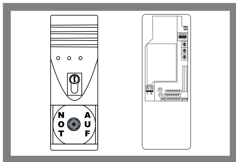
Fig. 1: Terminal de commande pour portedesecours1338- à droite, la face arrière ouverte
