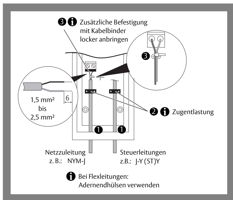
Abb. 2: Vorbereitende Arbeiten
