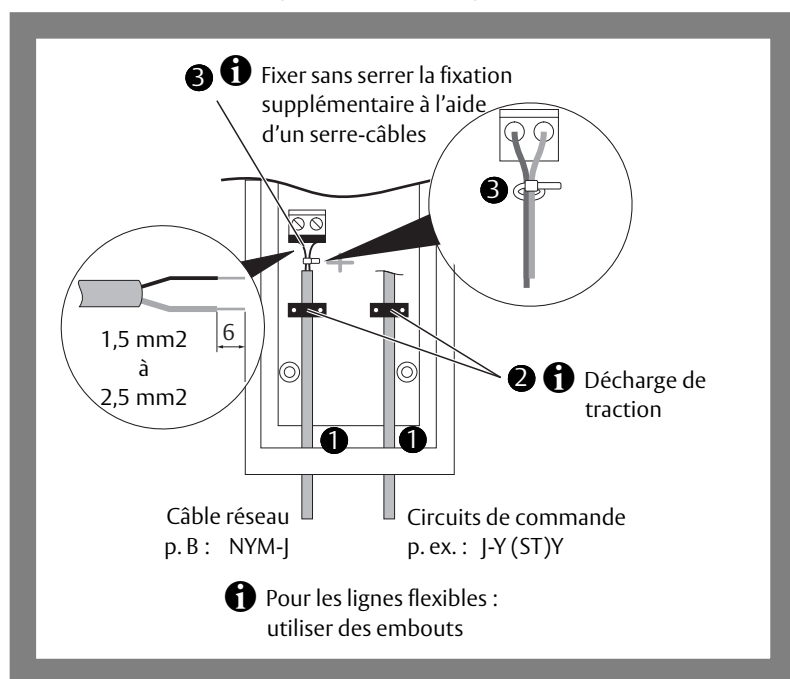
Fig. 2: Travaux préparatoires
