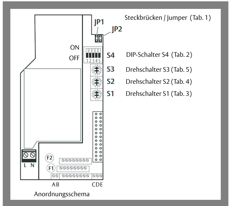
Abb. 7: Schaltelemente und Anschlüsse
