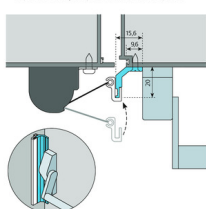
Variante de montage A Le profilé de montage LP1 passe directement devant le push bar
