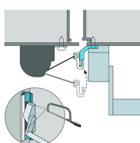
Variante de montage B Le profilé de montage LP1 est interrompu au push bar
